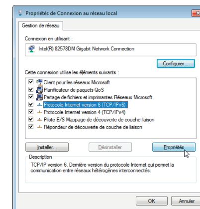
TCP/IPv6 sélectionné
