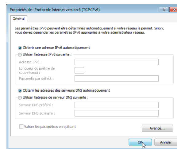
Propriétés TCP/IPv6
